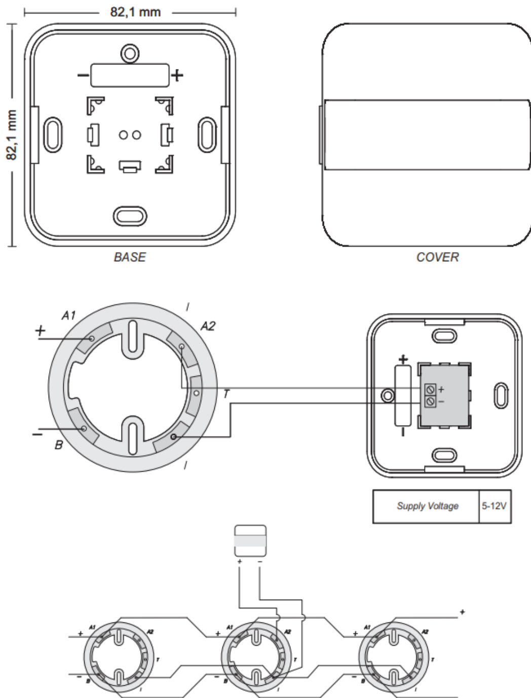
Példa több érzékelő azonos másodkijelzőre való kötésére
